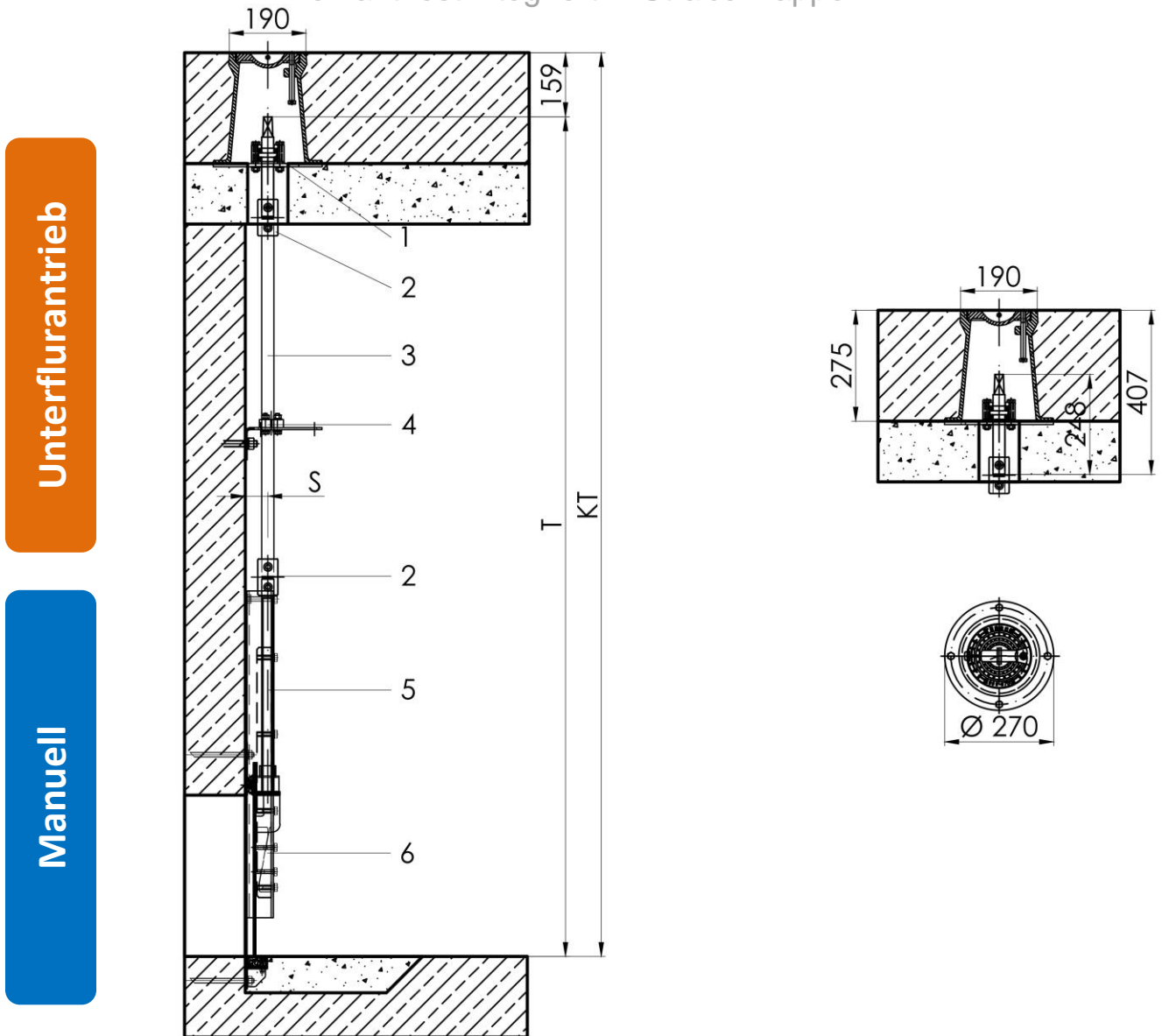
Einbausituation mit Schieber C20-Serie
