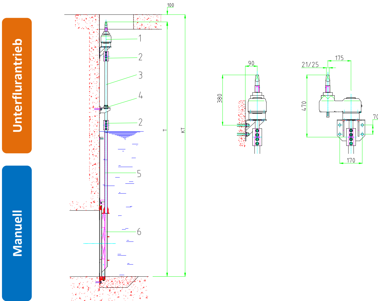
Einbausituation mit Schieber C20-Serie
