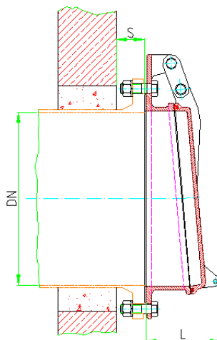
Flanschversion passend für bauseitigen Flansch DIN 2501 PN 10
