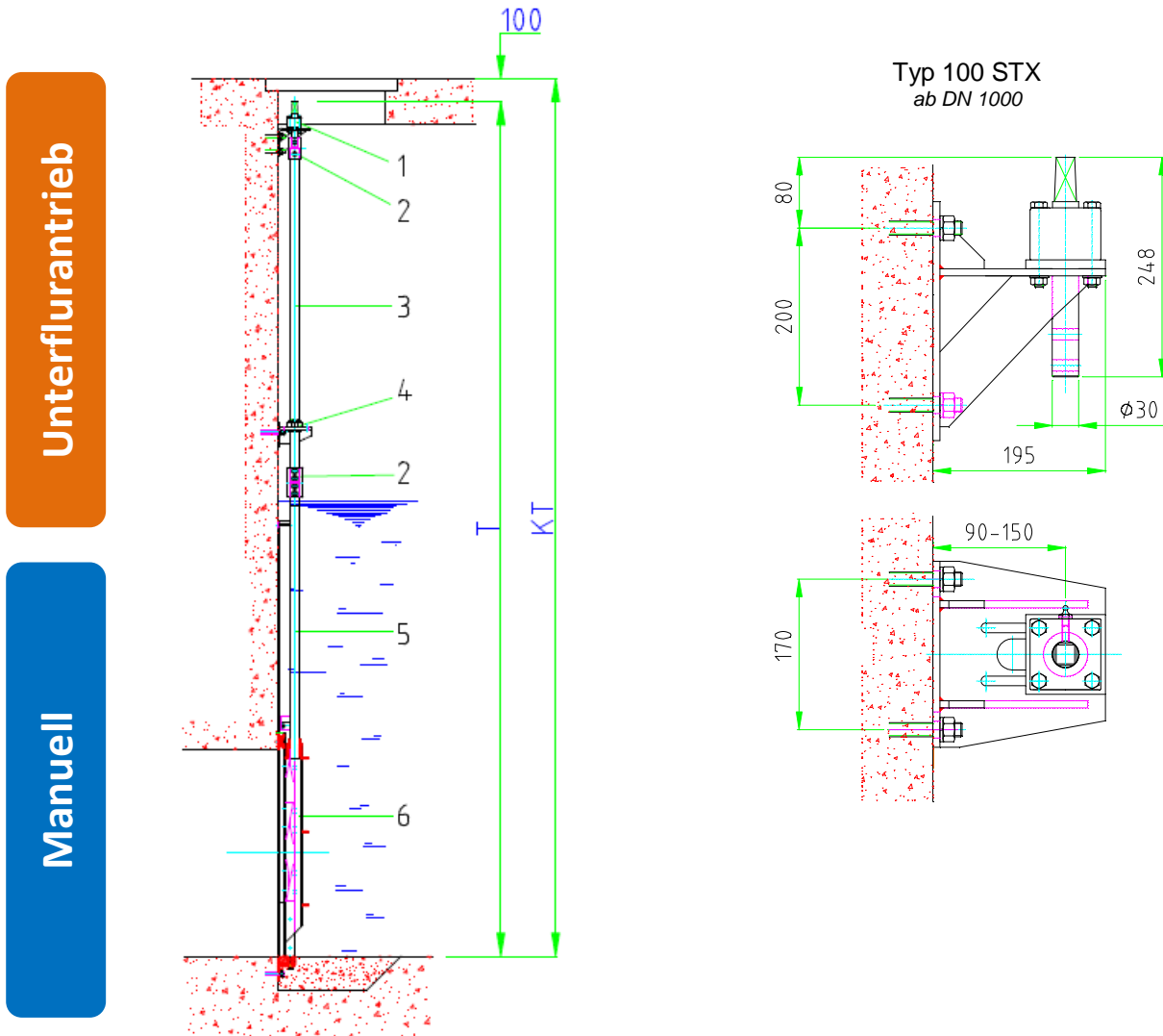
Einbausituation mit Schieber C20-Serie
