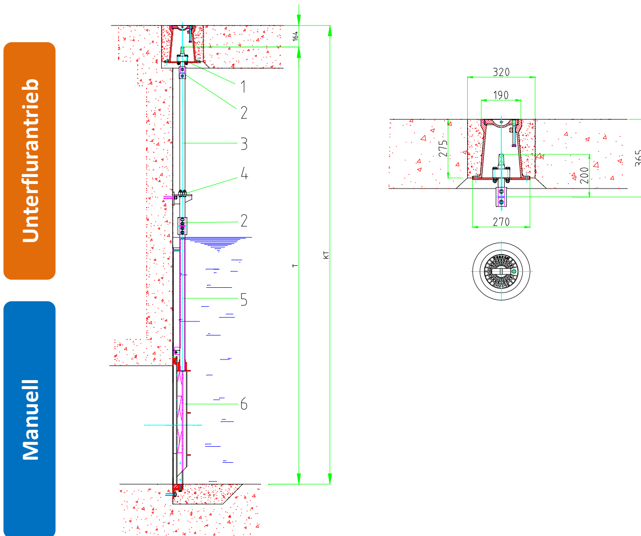
Einbausituation mit Schieber C20-Serie
