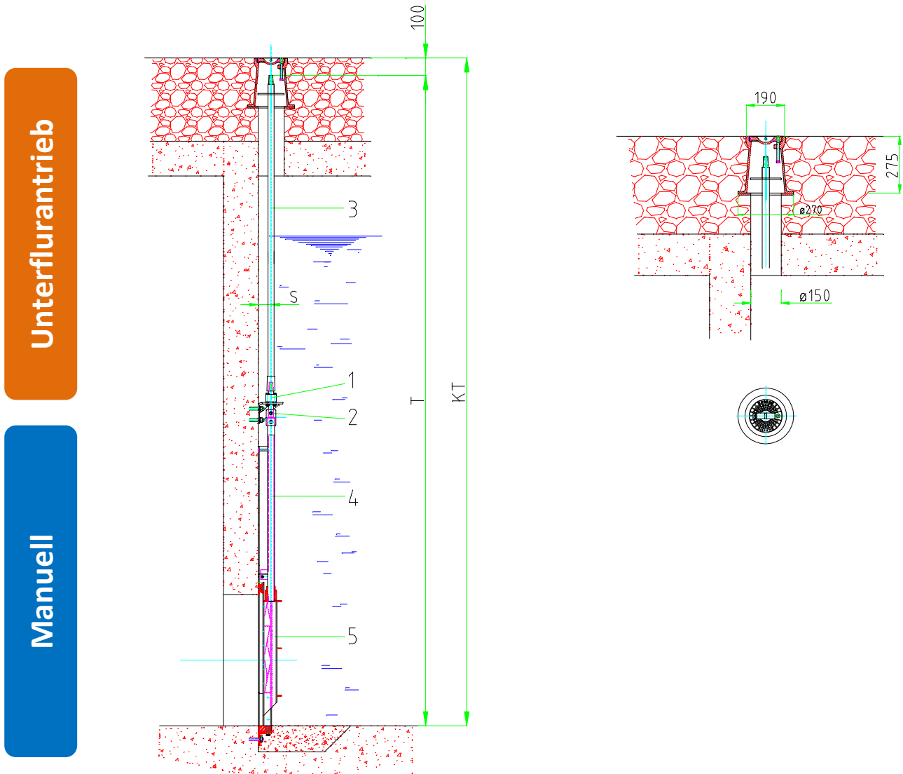
Einbausituation mit Schieber C20-Serie
