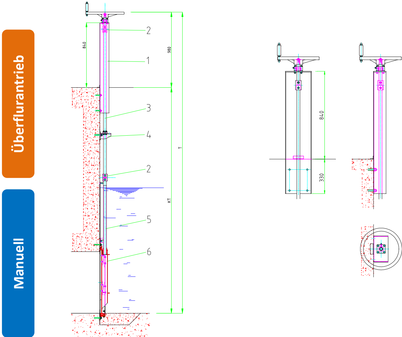
Einbausituation mit Schieber C20-Serie
