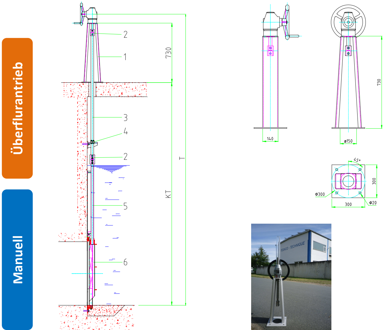
Darstellung mit Hubspindel und Schutzrohr
