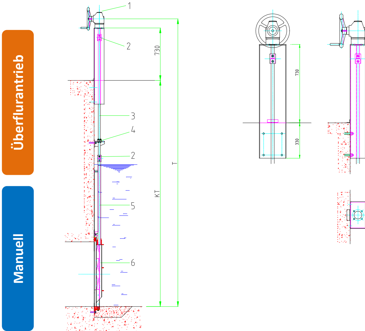
Einbausituation mit Schieber C20-Serie
