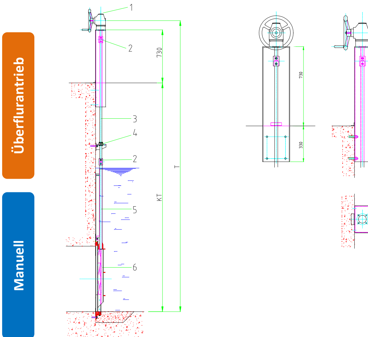
Einbausituation mit Schieber C20-Serie
