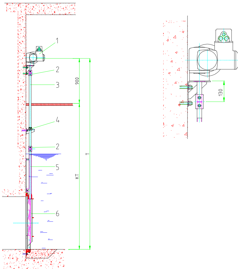
Einbausituation mit Schieber C20-Serie
