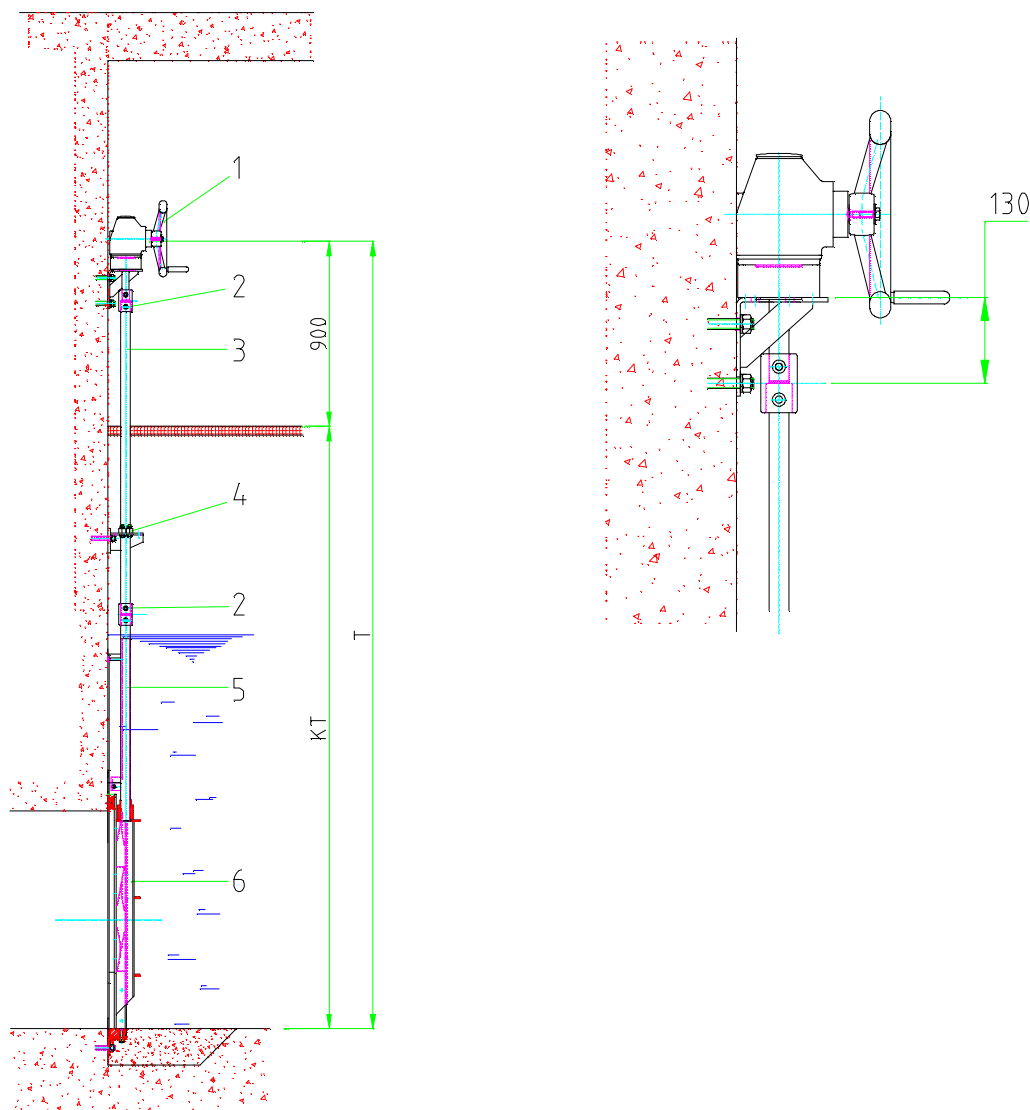
Einbausituation mit Schieber C20-Serie
