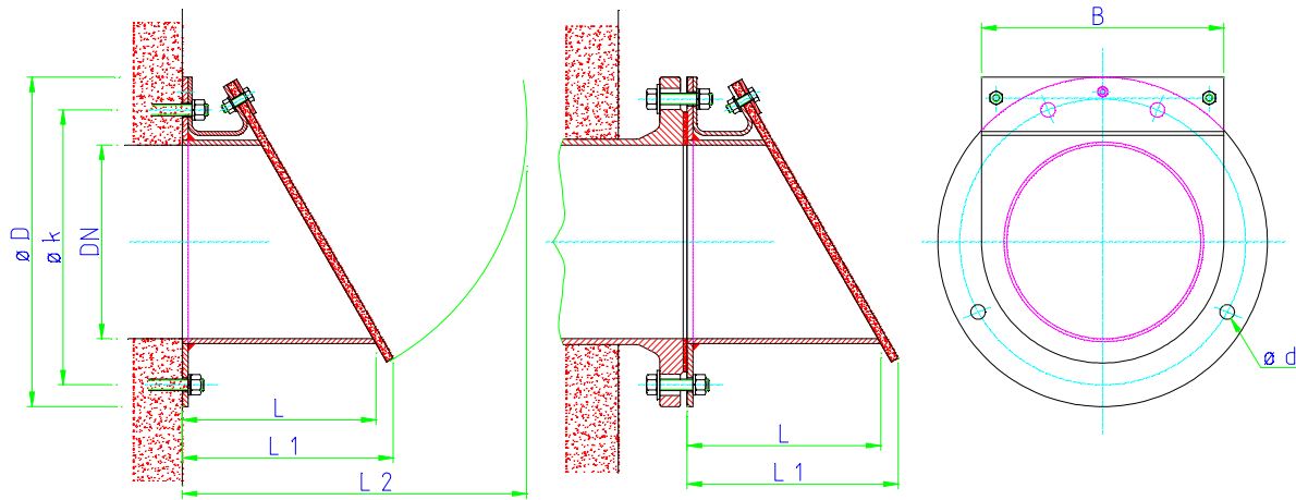
Dübelversion
