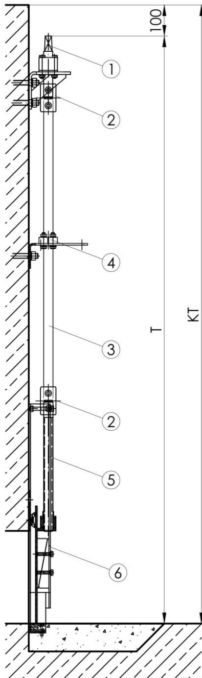
Einbausituation mit Schieber C20-Serie
