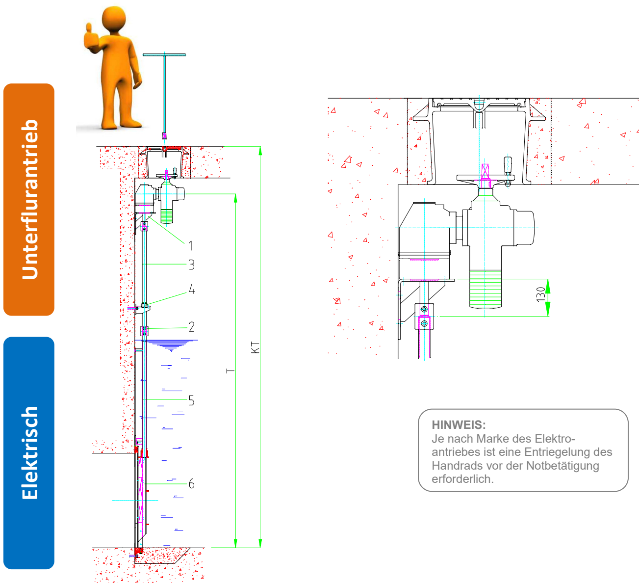
Einbausituation mit Schieber C20-Serie
