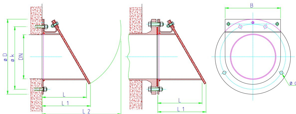
Dübelversion
