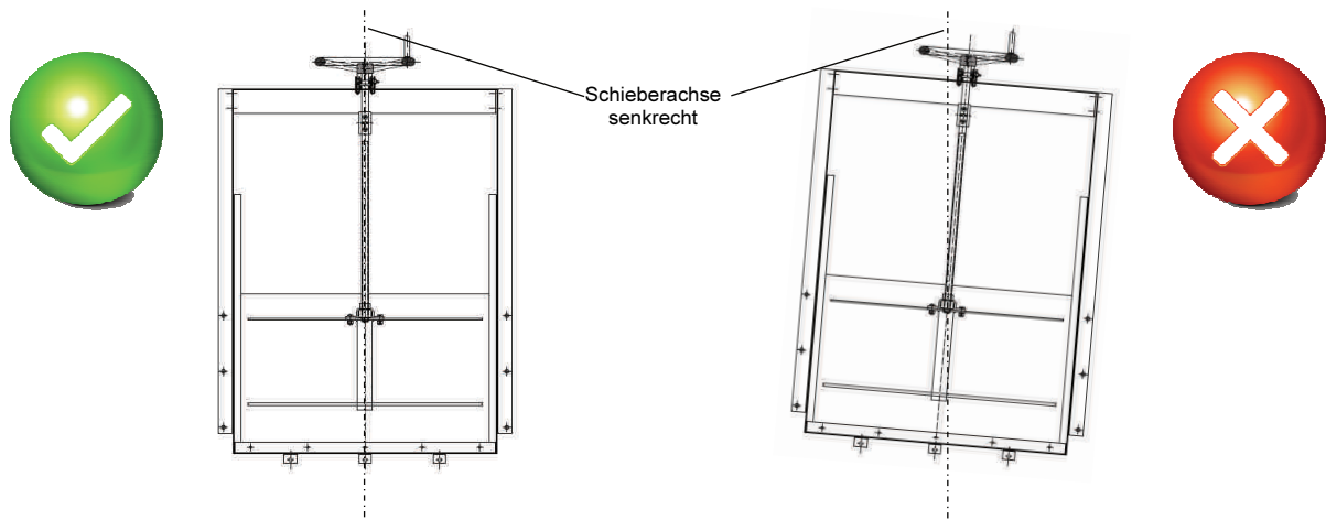
Fig. 2.4 - Senkrechter Einbau
