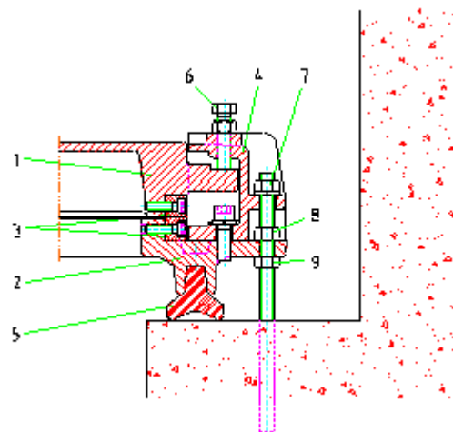
Fig. 3 - Setzen der Ankerstangen
