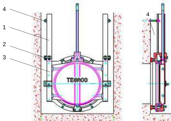
Fig. 4 - Seitenführungverlängerung
