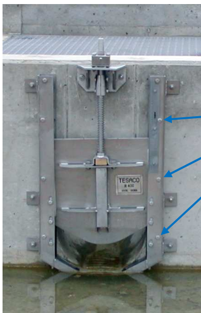
Fig. 1 - Darstellung Drosselschieber mit Gleitleisten
