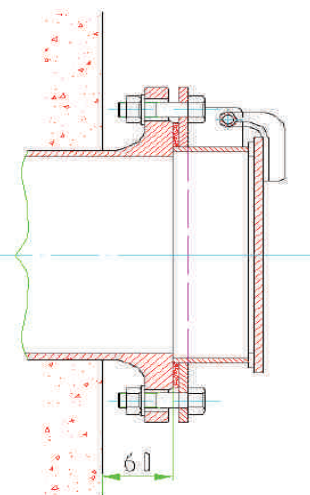
Flanschversion mit reduzierter Blattstärke, passend für bauseitigen Flansch DIN 2501 PN 10
