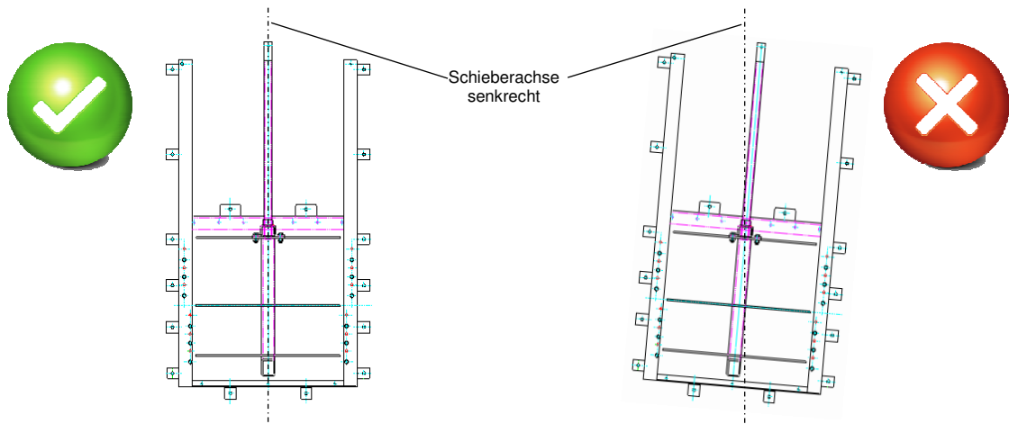
Fig. 2.5 - Senkrechter Einbau
