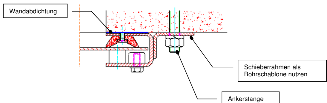
Fig. 3.4 - Setzen der Ankerstangen
